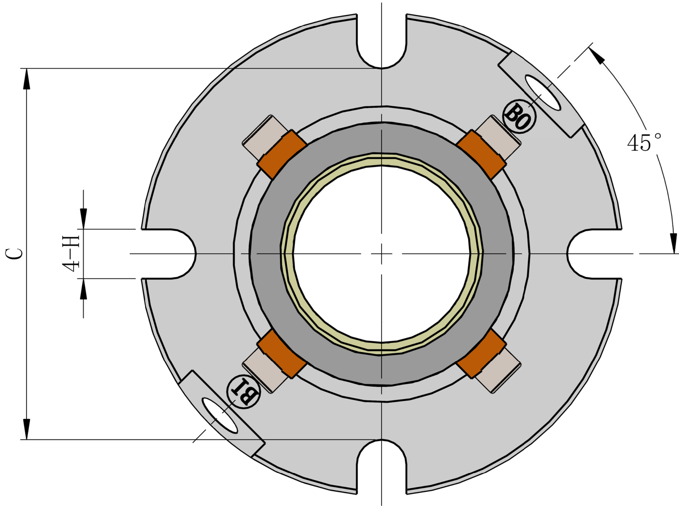
K向/View K 比例不符/NO SCALE
