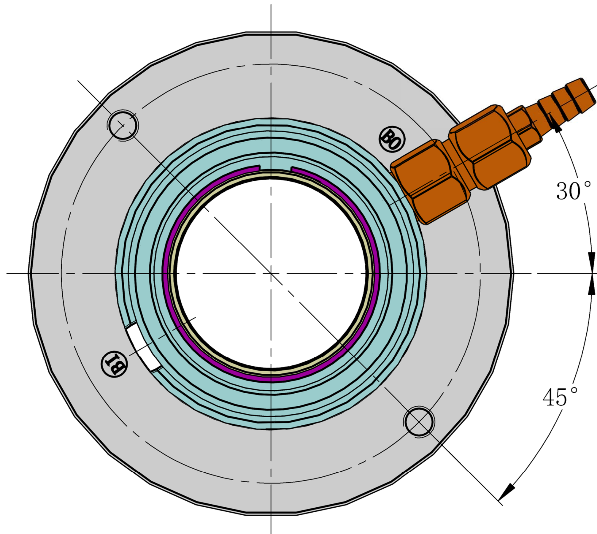
K向/View K 比例不符/NO SCALE
